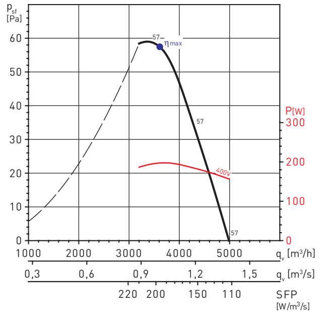
TCBT/6-500/H
